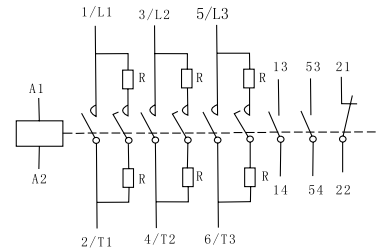
图1 示例CJ19-63/21、CJ19-95/21接触器内部连接图
